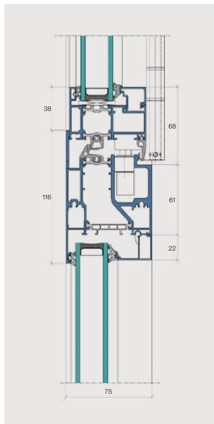
Coupe verticale IS-4000 sur allège IS-4
