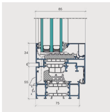
Coupe verticale fenêtre IS-4
