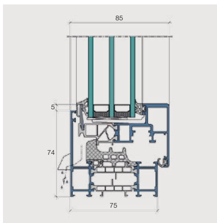
Coupe verticale fenêtre IS-4 à ouvrant caché
