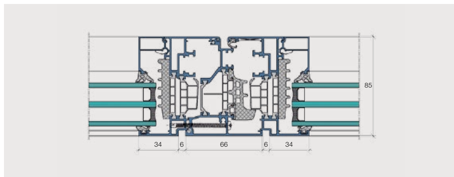
Coupe horizontale fenêtre IS-4 partie centrale (côte)
